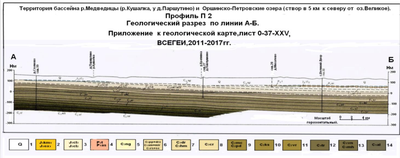
Рис. 33. Профиль П 2 (к рис.30). Геологический разрез по линии А-Б. Приложение к геологической карте, лист О-37-XXV. ВСЕГЕИ, 2011-2017 гг. [3]. Условные обозначения: 1 – четвертичные отложения; 2 – юрские отложения, нижнекиммержидский ярус и нижнеоксфордский подъярус, глины; 3 – верхнекевлловейский и среднекевлловейский подъярусы, глины; 4 – пермские отложения, татарский и ассельский ярусы, глины, алевроиты; отложения верхнего карбона: 5 – ногинская толща, доломиты; 6 – павлово-посадская и дрезнинская толщи, амеровская и малинниковская толщи, русавкинская и щелковская толщи, известняки мергели, глины; 7 – дорогомилловский и хамовнический горизонты, известняки, глины, мергели; 8 – кривякинский горизонт, известняки, мергели, глины; отложения среднего карбона: 9 – мячковский и подольский горизонты, известняки, доломиты, мергели; 10 – каширский горизонт, известняки, мергели, глины; 11 – верейский горизонт, глины; отложения нижнего карбона: 12 – протвинский, стешевский, тарусский горизонты, известняки, доломиты; 13 – веневский, михайловский горизонты, известняки, глины, алевроиты, пески; 14 – алексинский горизонт, глины, пески
