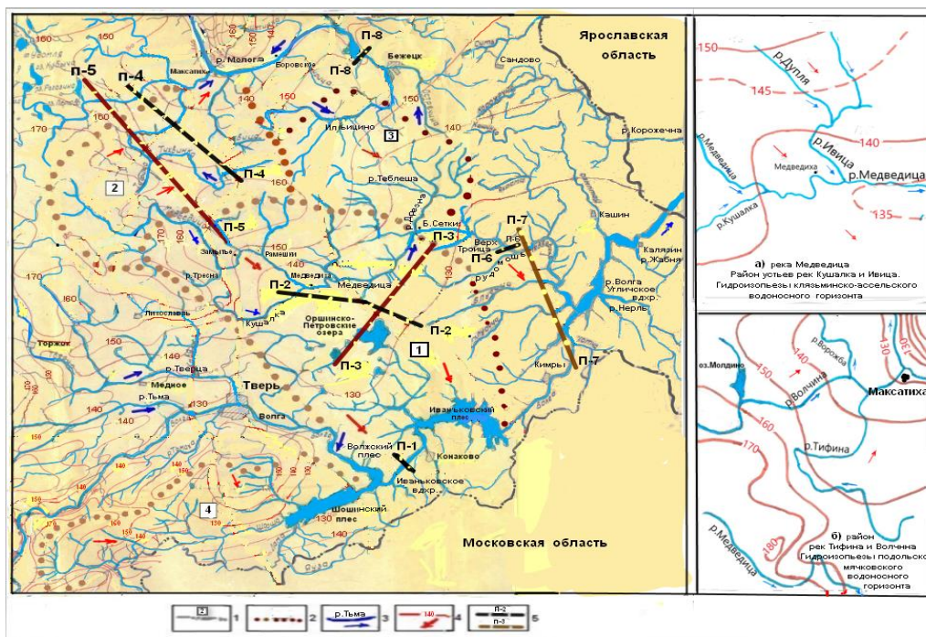
Рис. 30. Схема геологических и гидрогеологических разрезов по исследуемому району, с выделенными по гидроизопьезам подземными бассейнами: №1 – левобережная часть водосбора Волжского и Ивановского плесов Ивановского водохранилища; №2 – водосборы рек Тифины, Ривица; №3 – водосбор р.Дрезны; №4 – левобережная часть водосбора Шошинского плеса Ивановского водохранилища. Условные обозначения: 1 – граница Тверской области; 2 – граница подземных бассейнов, с указанием их порядкового номер, 3 – реки, озера; 4 – гидроизопьезы, вынесенные с Государственных гидрогеологических карт, М 1:200000; 5 – геологические профили, их порядковый номер, черный цвет – геологические разрезы (профили), коричневый цвет – геологические разрезы (профили) четвертичных отложений. Рисунки-вставки: а) гидроизопьезы клязьминско-ассельского водоносного горизонта в бассейне р. Медведица, район устьев рек Кушалка и Ивица. Взяты из гидрогеологической карты, лист 0-37-XXV, 1967г. [3]; б) гидроизопьезы подольско-мячковского водоносного горизонта в районе бассейнов рек Тифина и Волчина. Взяты из гидрогеологического отчета института ВНИГИК, Тверь, 1990г. [14]
